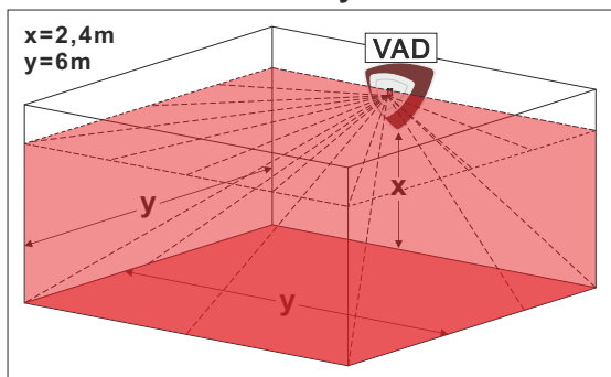
Σχήμα 1.Επιτοίχια Τοποθέτηση
